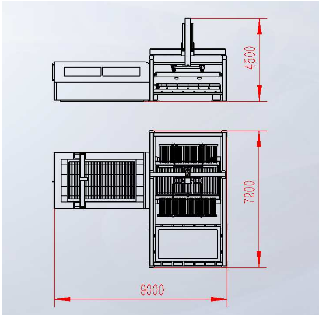
图 2-1 总装示意图
